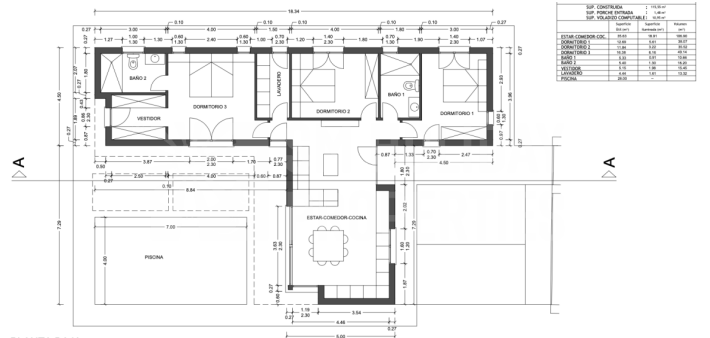
PLANTA BAJA COTAS Y SUPERFICIES
