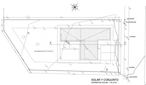
SOLAR Y CONJUNTO SUPERFICIE SOLAR: 716,19 m 2
